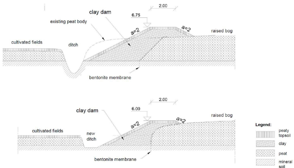
Figur 7-8 Skitse af dæmninger langs kant af højmosen: øverst på og nederst uden for den eksisterende moseflade (Fra Aalborg Kommune, udarbejdet til etablering langs Tofte Mose)
