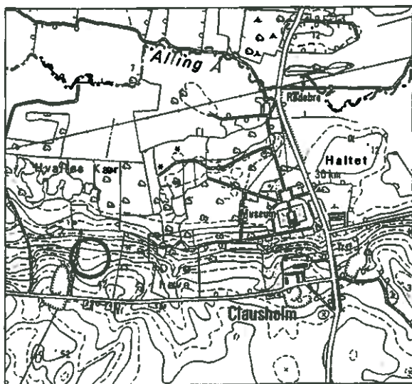
Fig. 48.1. Hvalløse. 1:25.000. Udsnit af kortblad 1315 III NØ (1985).
