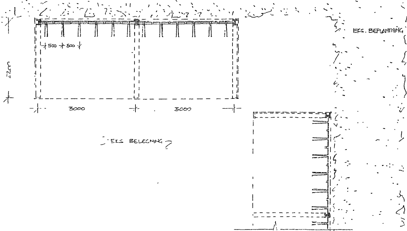
PLANSSNIT AF CYKELSKURE, MÅL 1:50
