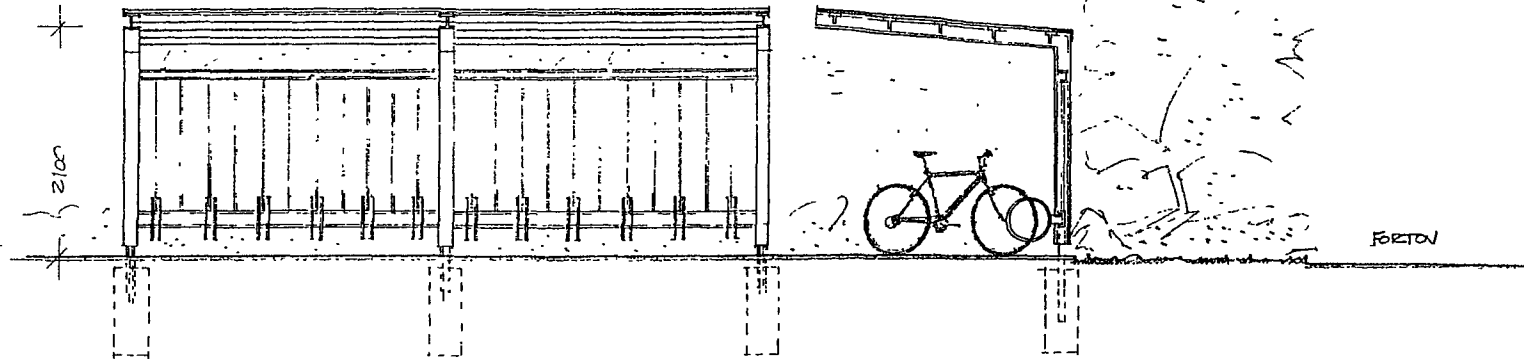
SNIT - OPSTALT AF CYKELSKURE, MÅL 1:50
