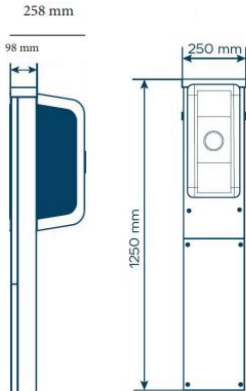
Sidebillede og opstalt af stander.
